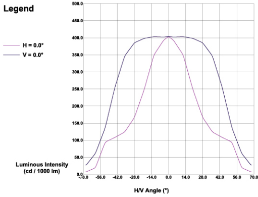
Iso-lux Diagram
